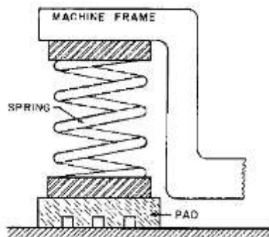
شکل خ-۴- فنر فلزی حمایت دار با لایه میراکننده یا نئوپرن یا دیگر الاستومر
