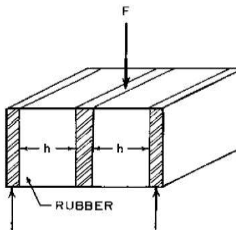
شکل خ-۲ - تحت برش بار مواد عایق بندی لاستیکی یا الاستومر ارتعاش
